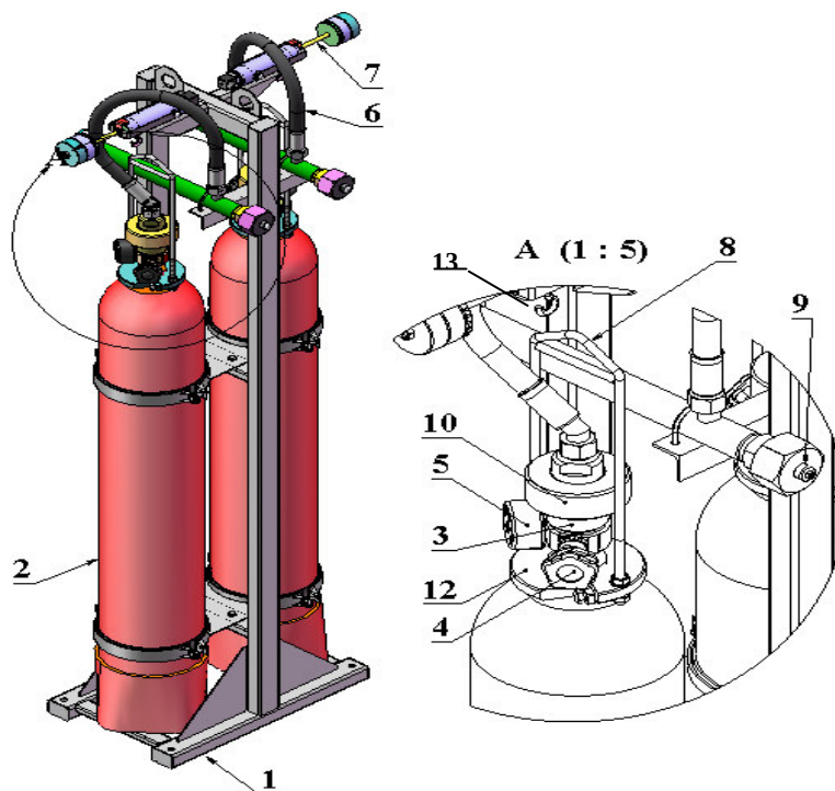
Рисунок-1. Секция дополнительная двухбаллонная 1 - рама; 2 - баллон; 3 - запорно-пусковое устройство; 4 – вентиль отсечной; 5 - манометр; 6 - рукав высокого давления; 7 - сигнализатор изменения массы; 8 - подвеска; 9 - клапан дренажный; 10 - груз контрольный; 11 - коллектор; 12 - кольцо; 13 - крюк.
