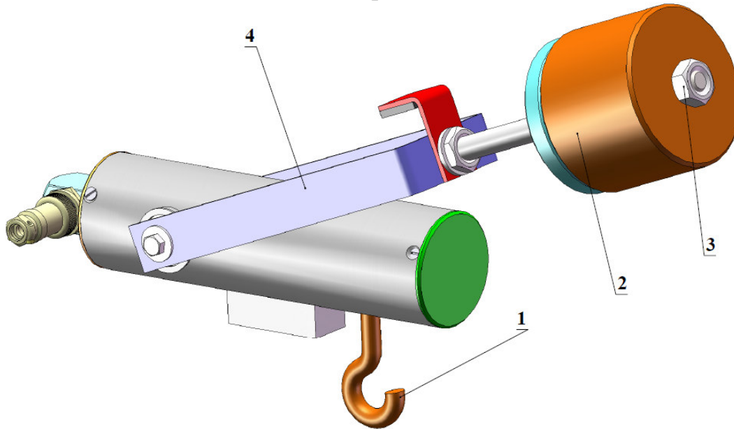
Рисунок-4. Сигнализатор изменения массы.
