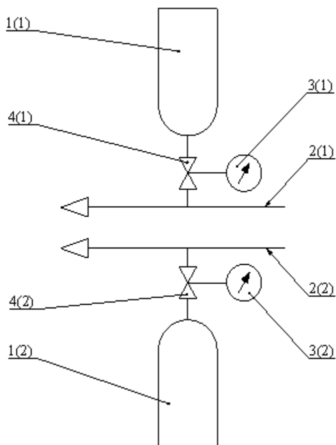
Рисунок-3. Секция дополнительная двухбаллонная Схема пневмогидравлическая принципиальная
